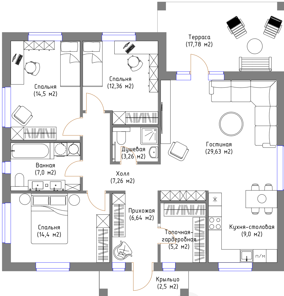
Проект дома «Ласточка» Планировка дома с возможной расстановкой мебели Общая площадь дома: 111,75 м 2
